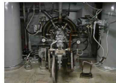
③ボイラ改造 (バーナ入替他)
