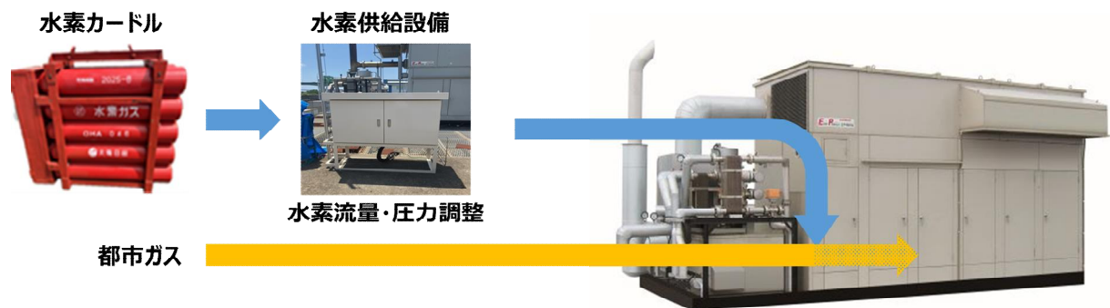
<水素混焼実証試験の設備フローイメージ>
