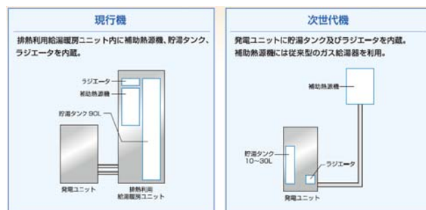
図 2 現行機および次世代機の構成
