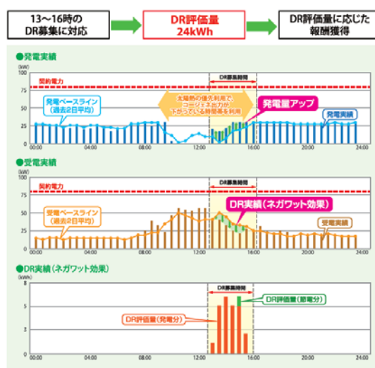
図3 コージェネによる DR 実証結果
