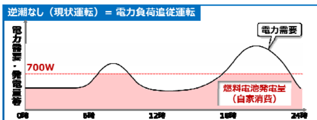
図 1 燃料電池(SOFC)の現状運転パターン
