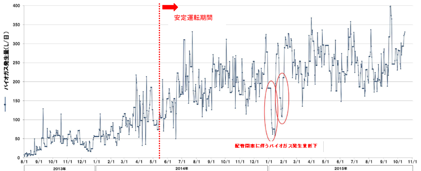
図 2 バイオガス発生量(日量)の推移
