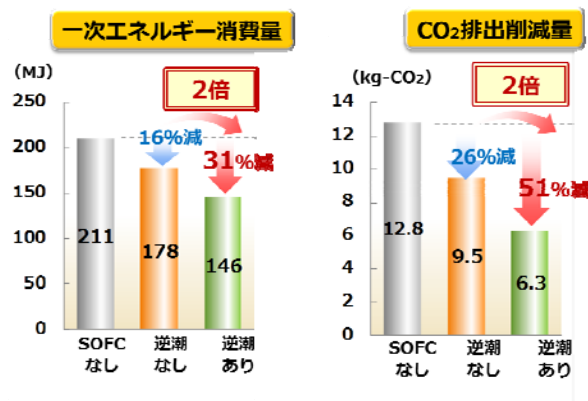
図 8 常時逆潮実施時の省エネ効果、CO 2 排出量削減効果
