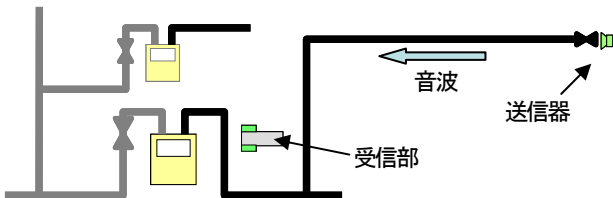
図1. 配管系統調査概念図
